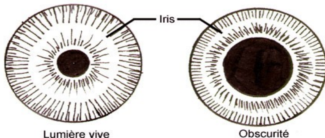
Variation de la pupille suivant l'éclairage
